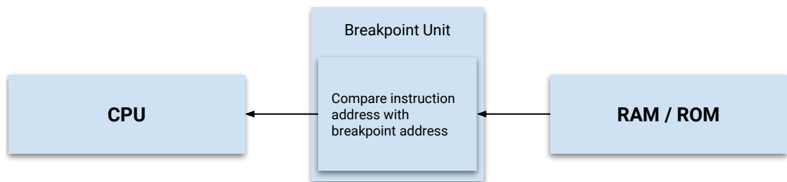
Abbildung 7.5.: Hardware Breakpoint Realisierung
